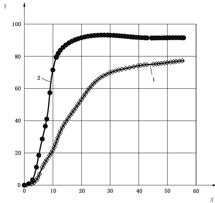
图 A.5 PLA 粉末(平均粒径 214.2 \mu\text{m} \pm 64.7 \mu\text{m} )依照 ISO 14855-2 中规定方法在 58 \text{ }^\circ\text{C} 时受控堆肥条件下的生物分解试验结果 [纤维素粉末(粒径尺寸 < 20 \mu\text{m} )作为阳性对照]
